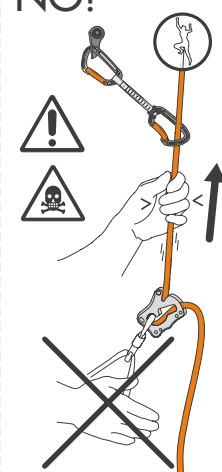
5.5 NO!
