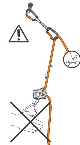
5.7 NO!
